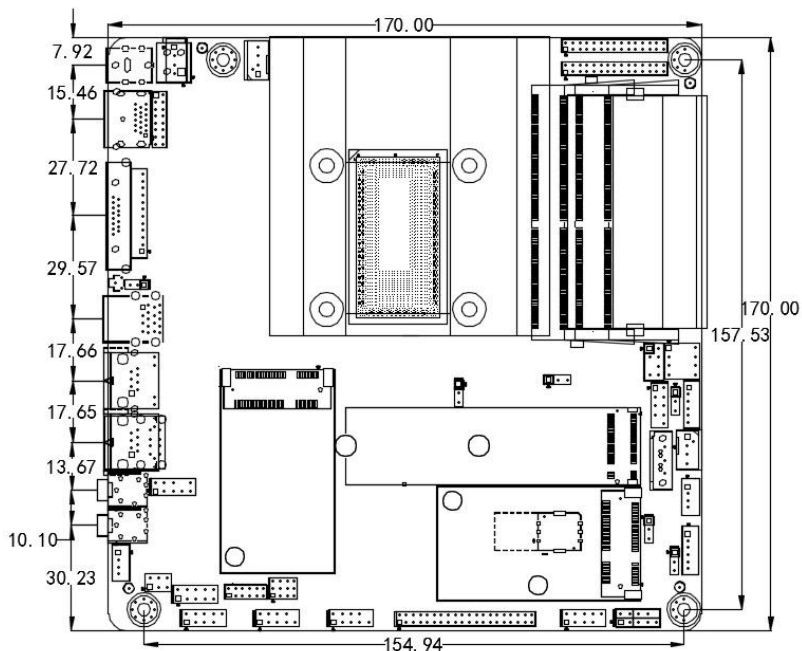
ITX-B100 VER:1.6尺寸图
