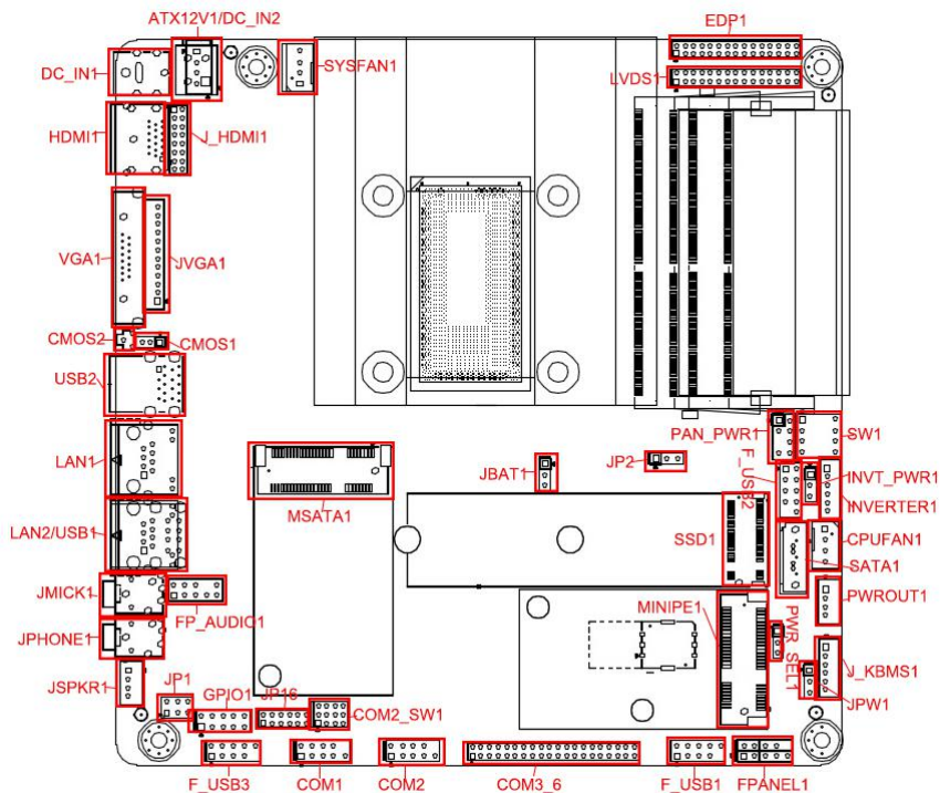
ITX-B100 VER:1.6 接口位置图
