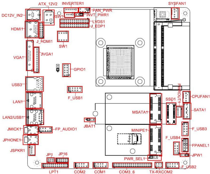
ITX-B346 接口位置图
