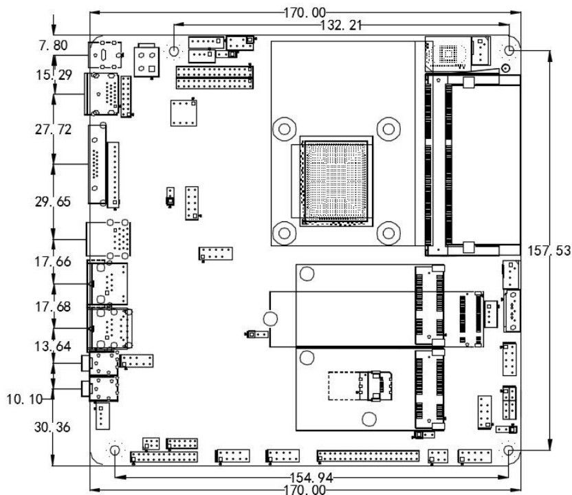
ITX-B346 VER:1.1 主板尺寸图
