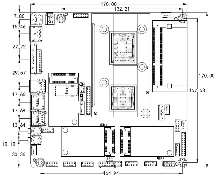
ITX-B320 VER:1.0 主板尺寸图
