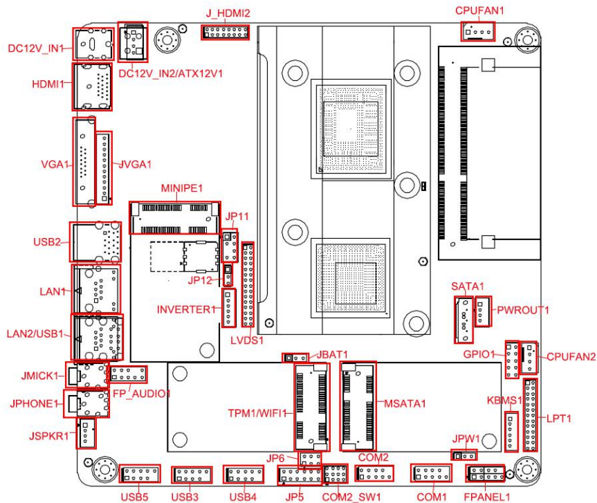
ITX-B320 接口位置图
