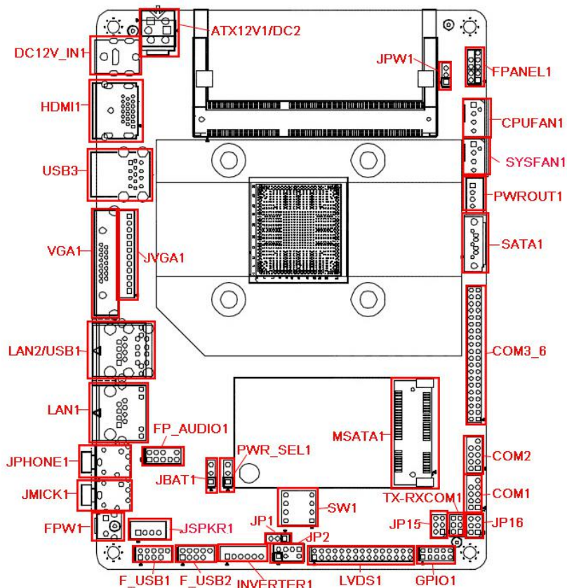
EPIC-N42 接口位置图
