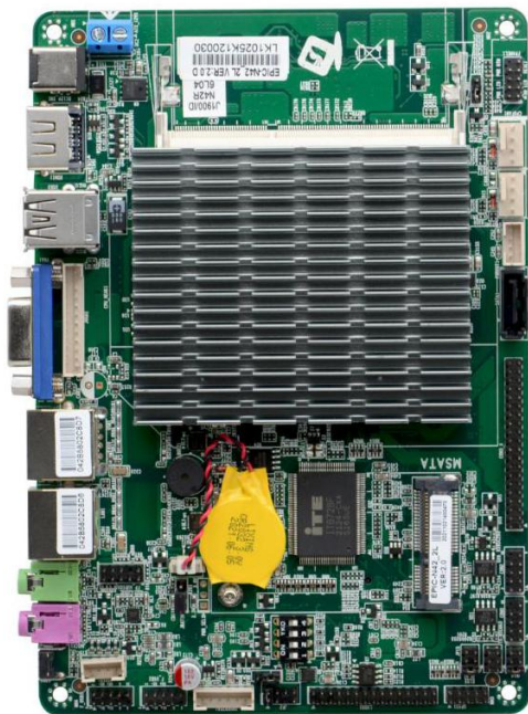
图一：EPIC-N42_2L VER:2.0 主板正面图
