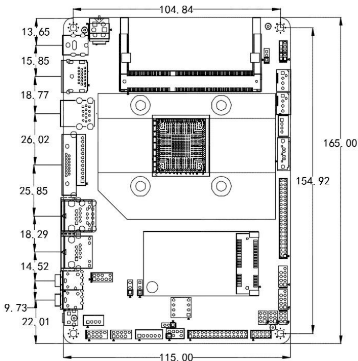
EPIC-N42 VER:2.0 主板尺寸图
