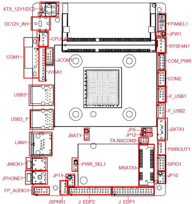
EPIC-A19 接口位置图
