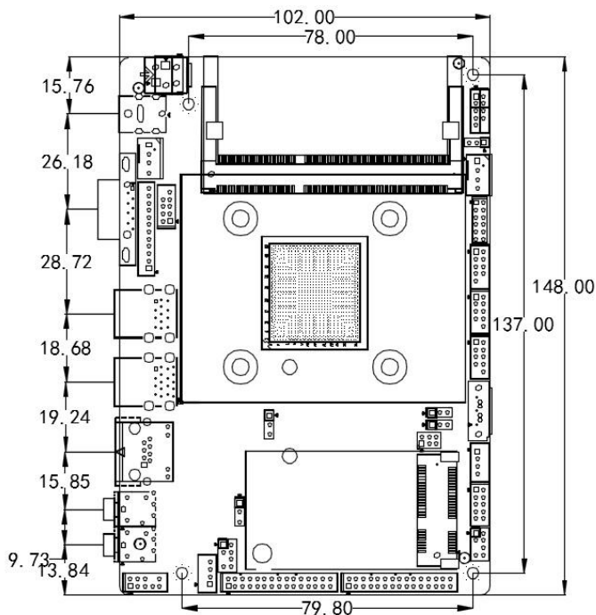
EPIC-A19 VER:1.1 尺寸图
